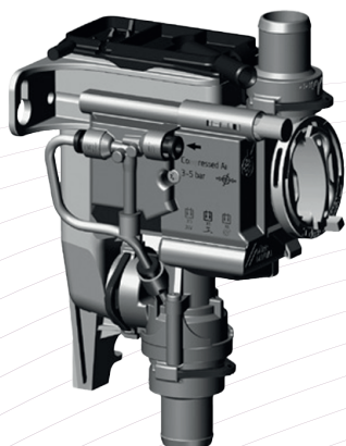
VANNE DE DRAINAGE DU CRACHOIR
