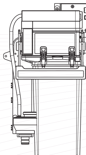
SÉPARATEUR AIR/EAU
